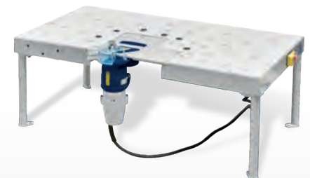
Abb. zeigt Kantenfräse KF 6 angebaut an Stationärtisch (KF 6 nicht im Lieferumfang enthalten)
