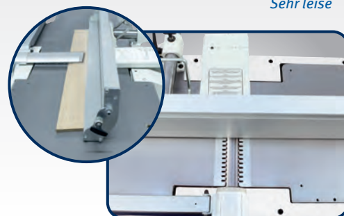
Abrichtanschlag · Stabiler, großer Abrichtanschlag aus Aluminium (1200 x 160 mm) mit Hilfsanschlag · Präzise Rundstangenführung
