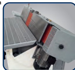
▶ Schleifaggregat per Handkurbel um 45° schwenkbar
